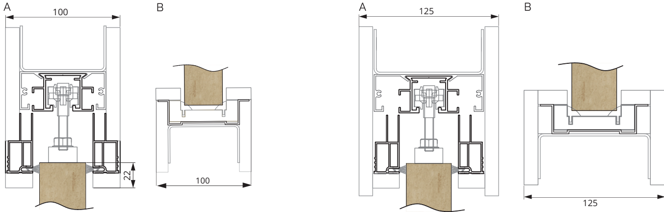
ZABUDOWA W ŚCIANIE 100 MM
