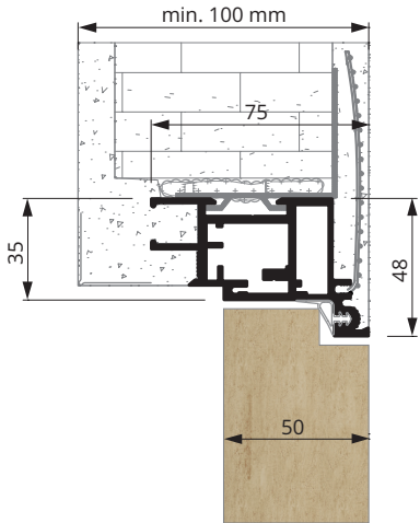
ZABUDOWA W ŚCIANIE MUROWANEJ
