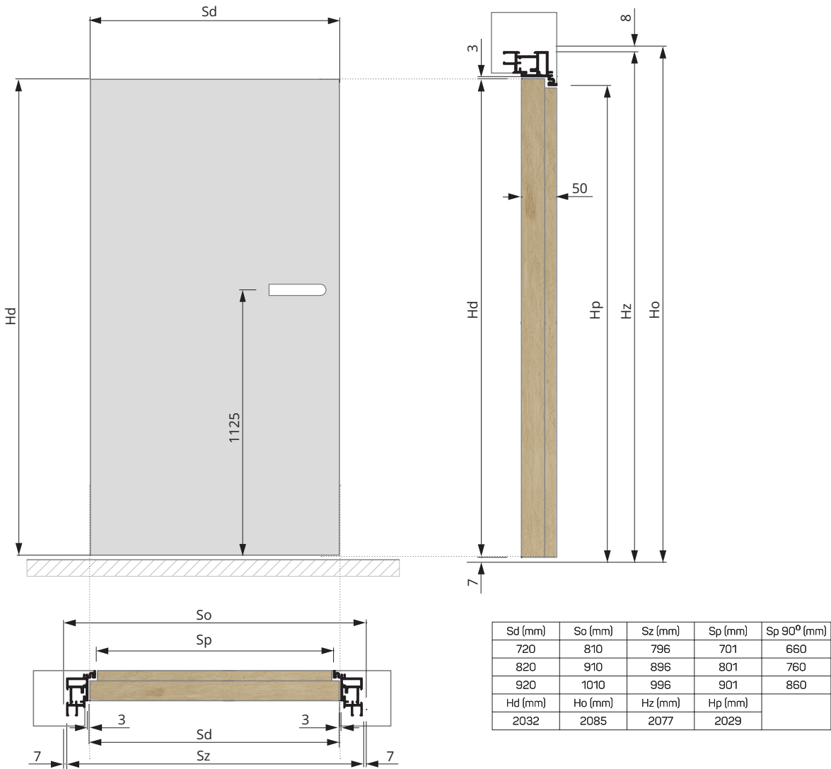
ZABUDOWA W ŚCIANIE MUROWANEJ
