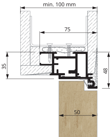
ZABUDOWA W ŚCIANIE GK
